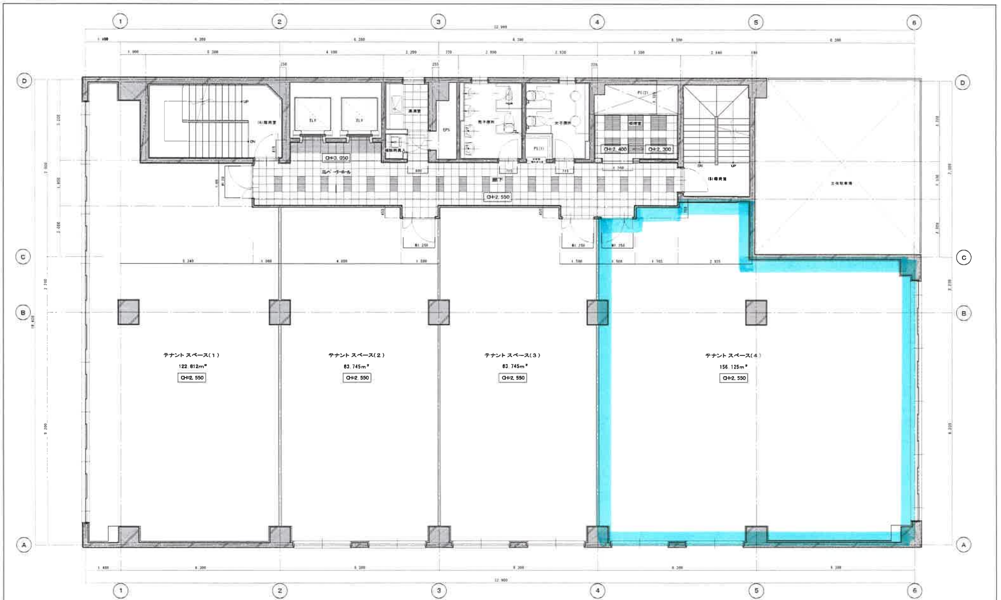
6 階 平 面 図 1:50
